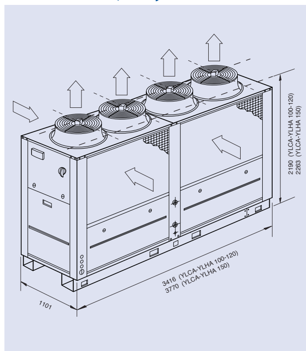
YLCA-YLHA 100, 120 y 150 T-TP
