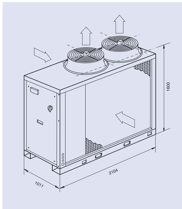
YLCA-YLHA 50 y 60 T-TP
