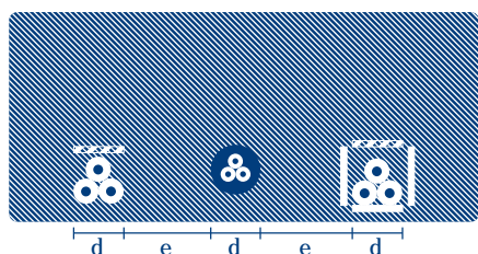
FIG. 4.1 – DESENHO ESQUEMÁTICO DA DISTRIBUIÇÃO DOS CABOS
