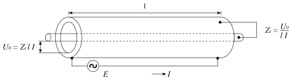
FIG. 1.5 – ESQUEMA ILUSTRATIVO DA IMPEDÂNCIA DE TRANSFERÊNCIA
