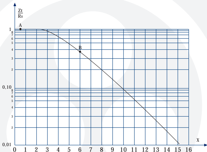
FIG. 1.6 – Curva típica da impedância de transferência de um cabo.
