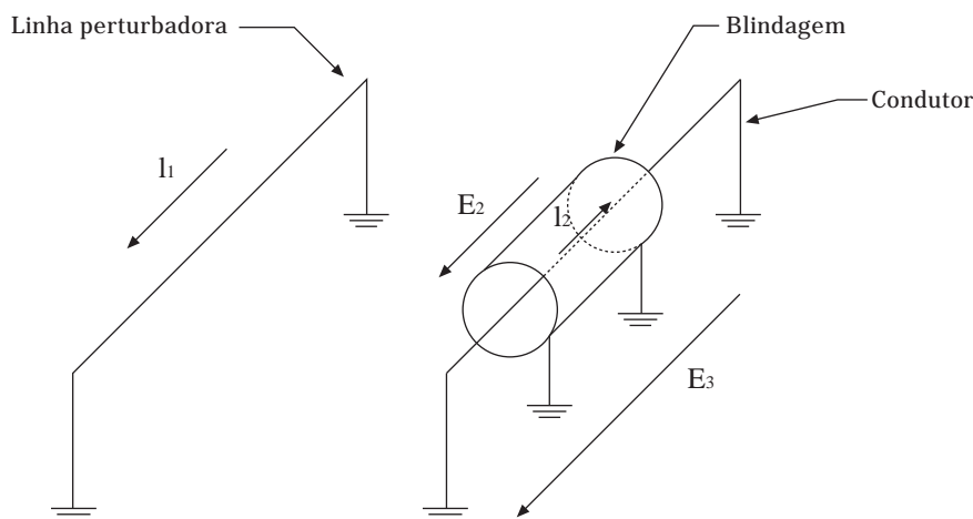
FIG. 1.7 – ILUSTRAÇÃO DA INFLUÊNCIA DA LINHA DE ENERGIA SOBRE O CONDUTOR E BLINDAGEM
