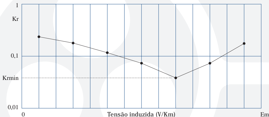
FIG. 1.8 – CURVA DO FACTOR REDUTOR PARA UM TIPO DE CABO
