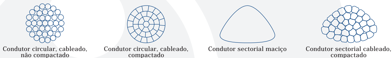
FIG. 1.1 - SECÇÃO RECTA TRANSVERSAL DE VÁRIOS TIPOS DE CONDUTORES
