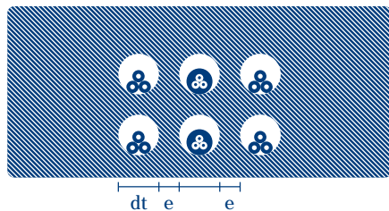
FIG. 4.2 – DESENHO ESQUEMÁTICO DA DISTRIBUIÇÃO DOS CABOS
